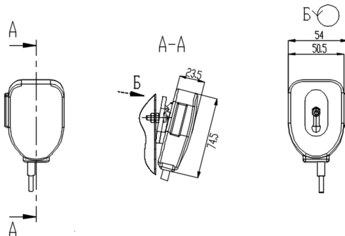
Рисунок 1 - Габаритный чертеж внешнего микрофона ВМ-03
